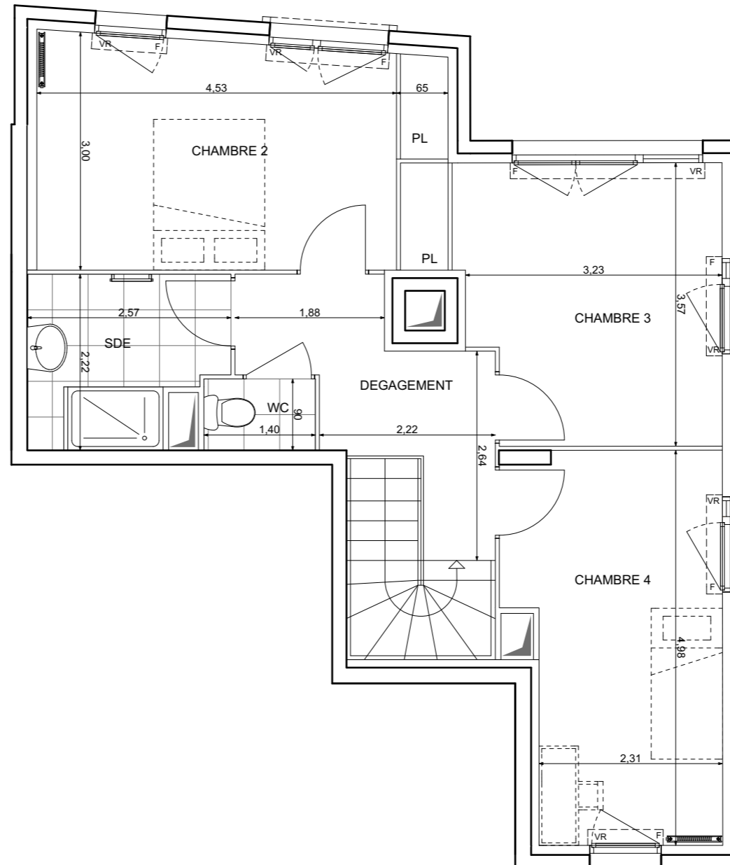
NIVEAU HAUT DE DUPLEX SURFACE HABITABLE 51,03 m 2
