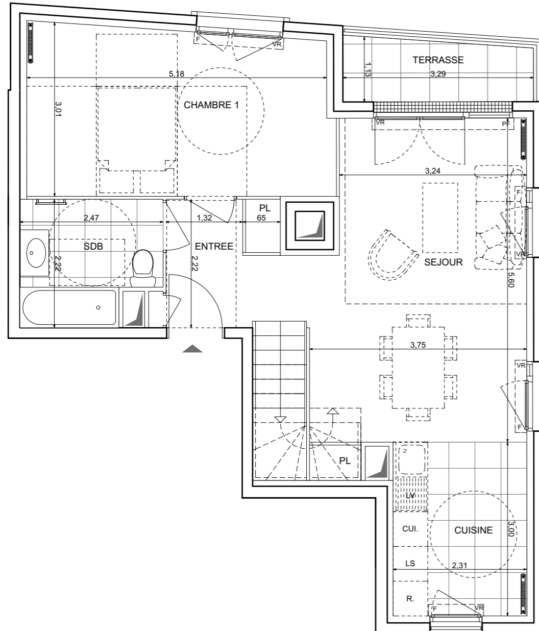
NIVEAU BAS DE DUPLEX SURFACE HABITABLE 51,98 m 2
